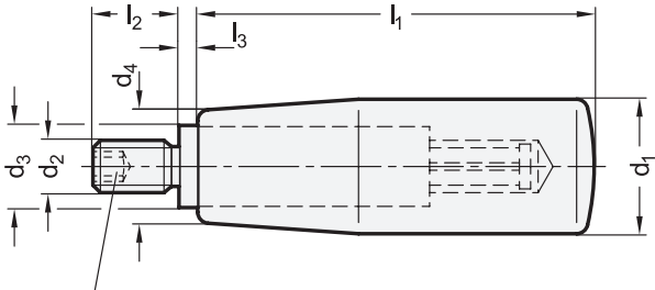
Gniazdo sześciokątne
